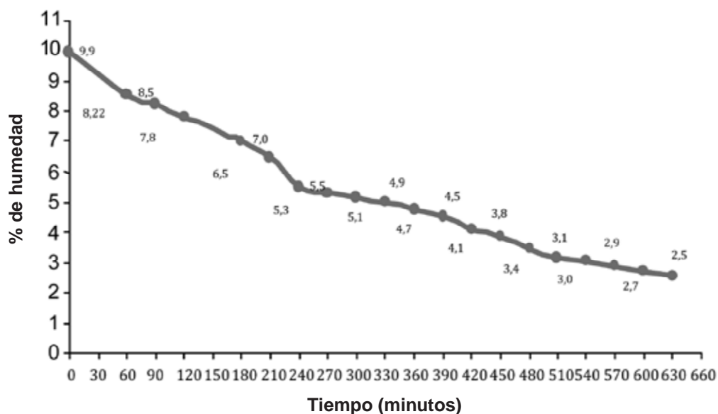
Figura 1. Curva de secado de semillas de tomate (Relación Silica - Semilla de 5.1)
