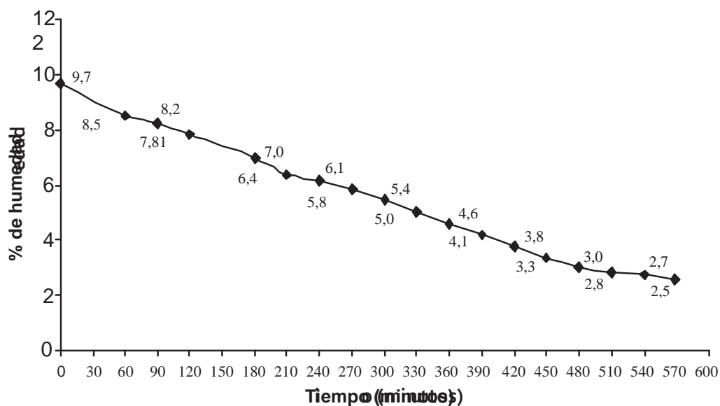
Figura 2. Curva de secado de semillas de pimentón (Relación Silica - Semilla de 5:1)
