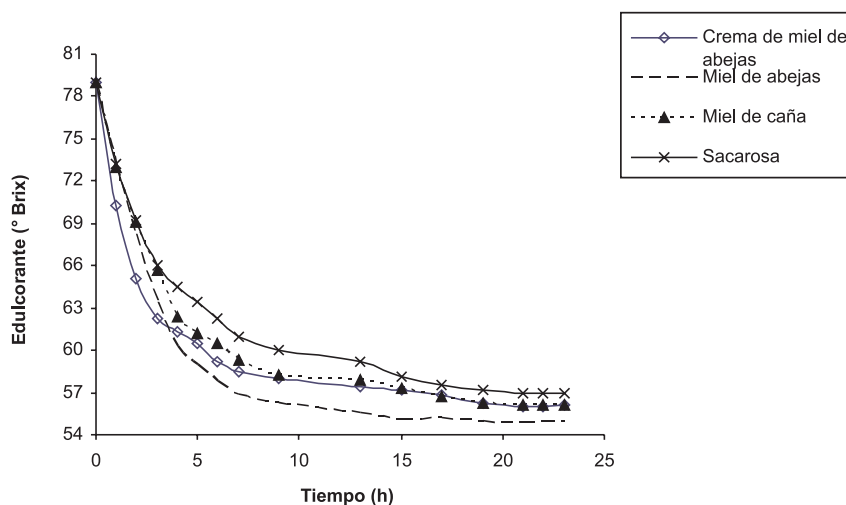
Figura 2. Tendencia cinética de los diferentes agentes edulcorantes utilizados para la deshidratación osmótica de papaya hawaiana.
