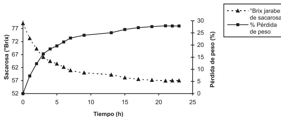
Figura 3. Comportamiento de los °Brix del edulcorante sacarosa y el peso de frutos de papaya hawaiana, sometidos a deshidratación osmótica.
