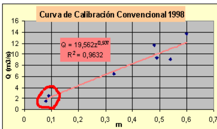
Figura 10.2. Curva de calibración convencional río Supía 1998
