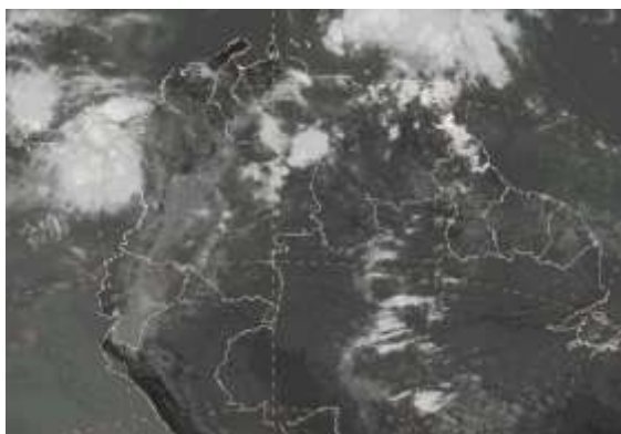
Figura 3.8. Centro de baja presión semipermanente del Golfo de Panamá. Fuente: NASA, http://weather.msfc.nasa.gov/GOES
