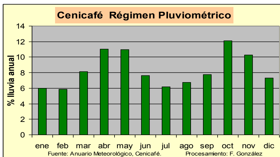
Figura 3.4. Régimen Pluviométrico Ecuatorial Perfecto
