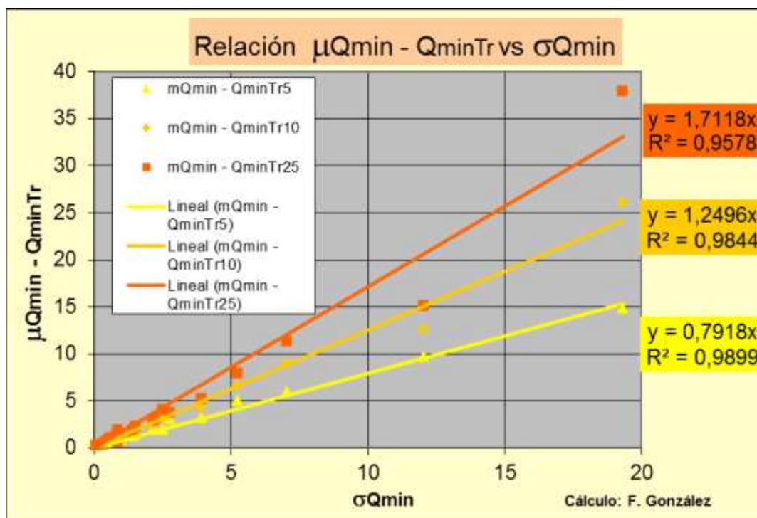
Figura 10.18. Relaciones \mu Q_{min} - Q_{minTr} vs \sigma Q_{min} .
