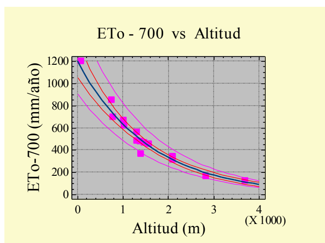
Figura 7.1 Ajuste del modelo de regresión exponencial ETo vs altitud.
