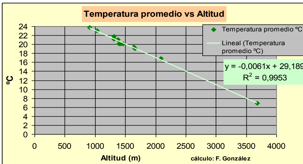
Figura 4.1. Temperatura promedio (°C) vs Altitud (m). 39
