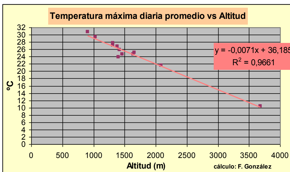
Figura 4.3. Temperatura máxima diaria promedio (°C) vs Altitud (m).
