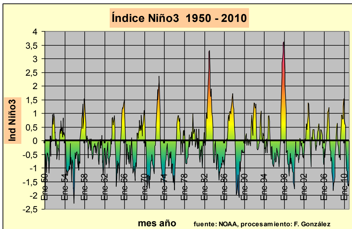
Figura 3.22. Índice Niño3 1950 – 2010.
