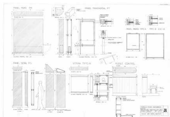
Plano de una sección del mobiliario museográfico diseñado por Carlos Niño para el Museo Siderúrgico de Acerías Paz del Río. Carlos Niño; 1981. Archivo Carlos Niño.
