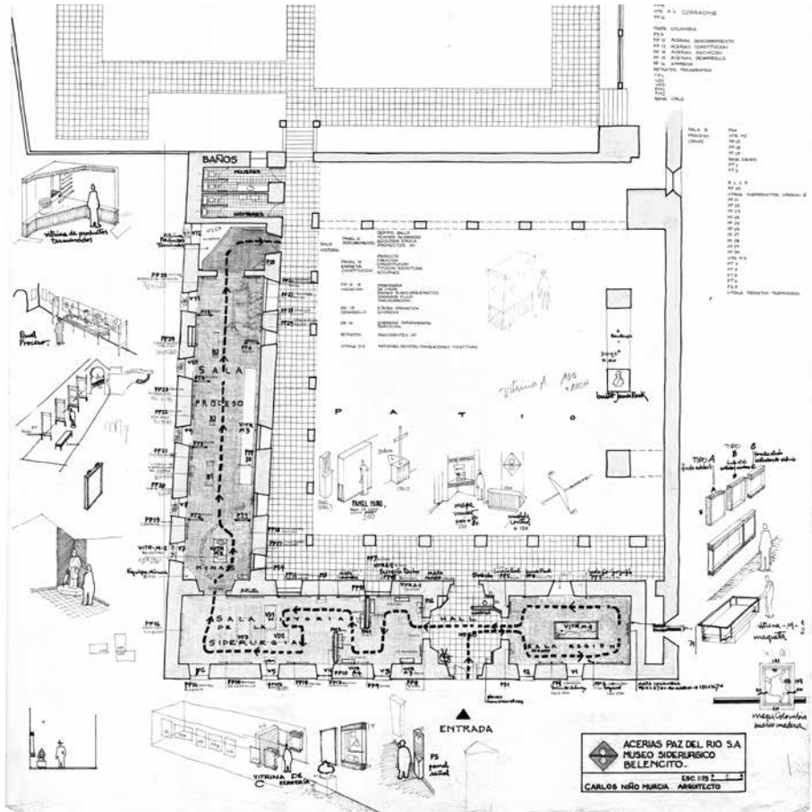
Plano general de la exposición permanente del Museo Siderúrgico de Acerías Paz del Río. Carlos Niño; 1981. Archivo Carlos Niño.
