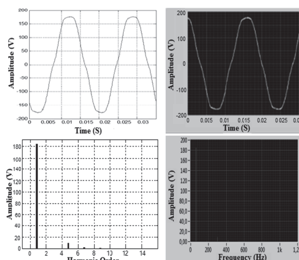
Figura. 16. Forma de onda y espectro en Matlab y Labview. Fuente: Autores.
