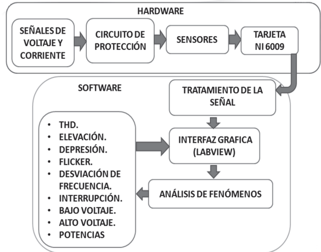
Figura. 2. Estructura del sistema. Fuente: Autores.
