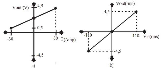
Figura.4 Escalonamiento de las señales. Fuente: Autores.
