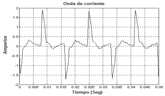
Figura 20. Forma de onda de corriente de la carga no lineal. Fuente: Autores.
