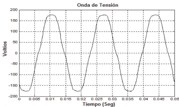
Figura 19. Forma de onda de tensión con la carga no lineal. Fuente: Autores.
