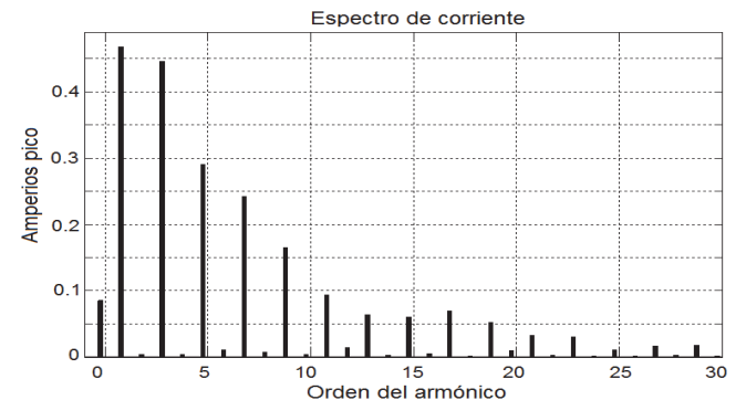
Figura 22. Espectro de la onda de corriente. Fuente: Autores.
