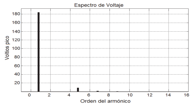
Figura 21. Espectro de la onda de tensión. Fuente: Autores.
