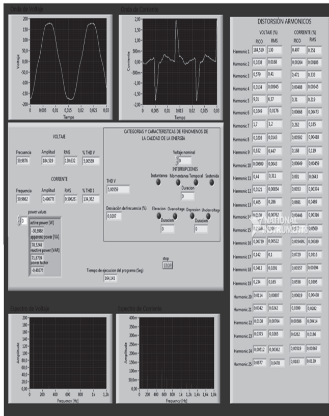
Figura 18. Resultados del sistema para la carga no lineal. Fuente: Autores.
