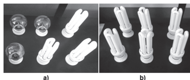
Figura 17. a) Carga mixta. b) Carga no lineal. Fuente: Autores.
