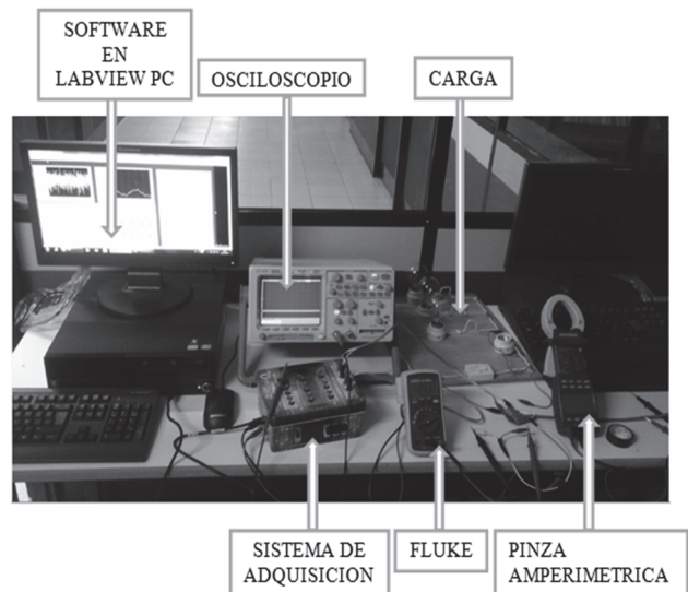
Figura. 13. Fotografía prueba de validación. Fuente: Autores.
