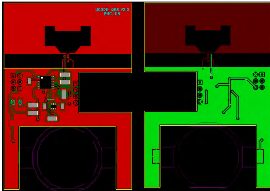
Figura 3-8. PCB del prototipo.
