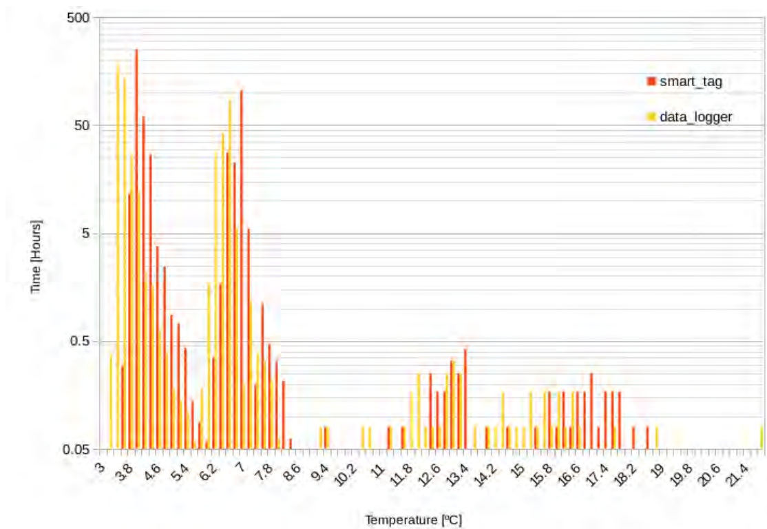
Figura 4-5. Temperatura registrada en calabaza troceada.
