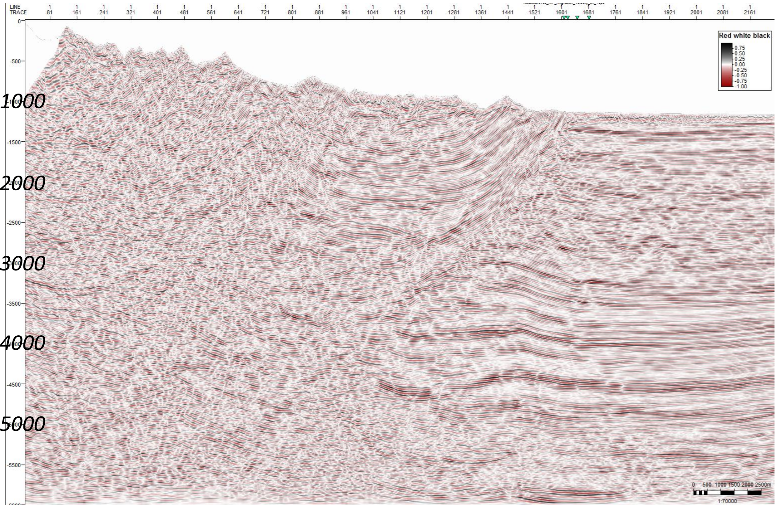
G Anexo: Sección sísmica Migrada y Post Apilada en tiempo PostSTM.
