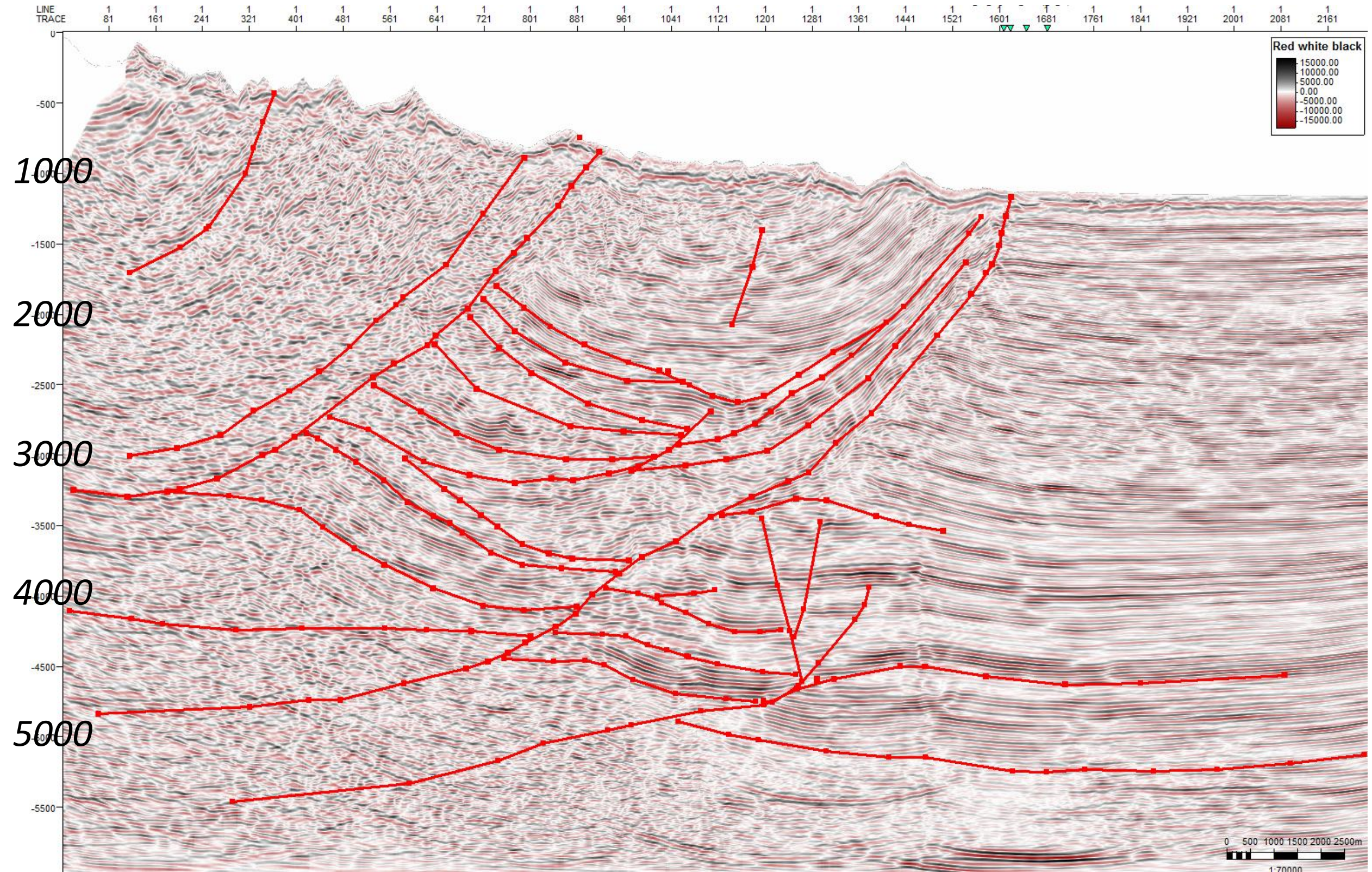
K Anexo: Sección sísmica Post Apilada Multifoco con interpretación geológica.
