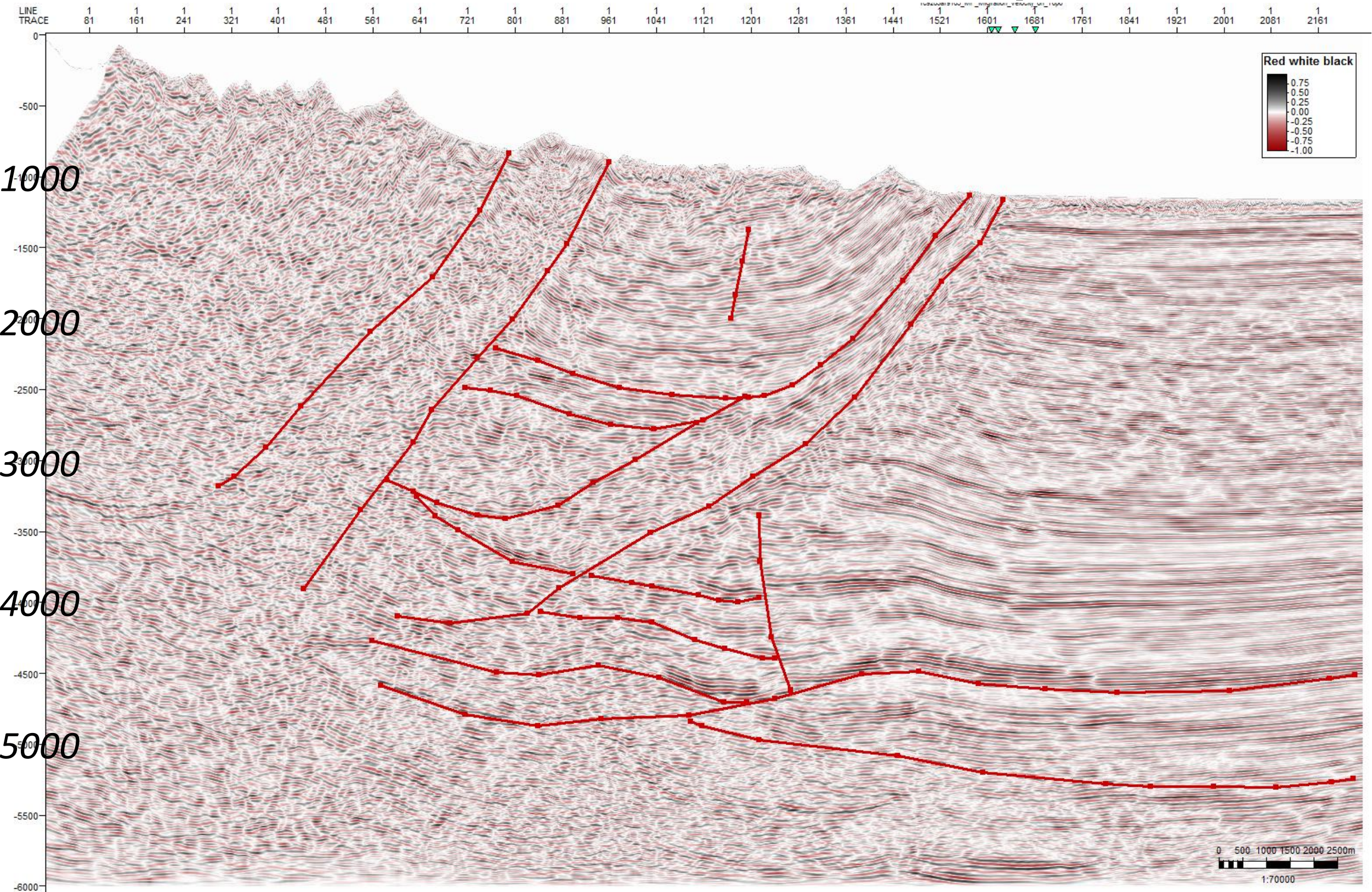
J Anexo: Sección sísmica Migrada y Post-apilada en tiempo PostSTM con interpretación geológica.
