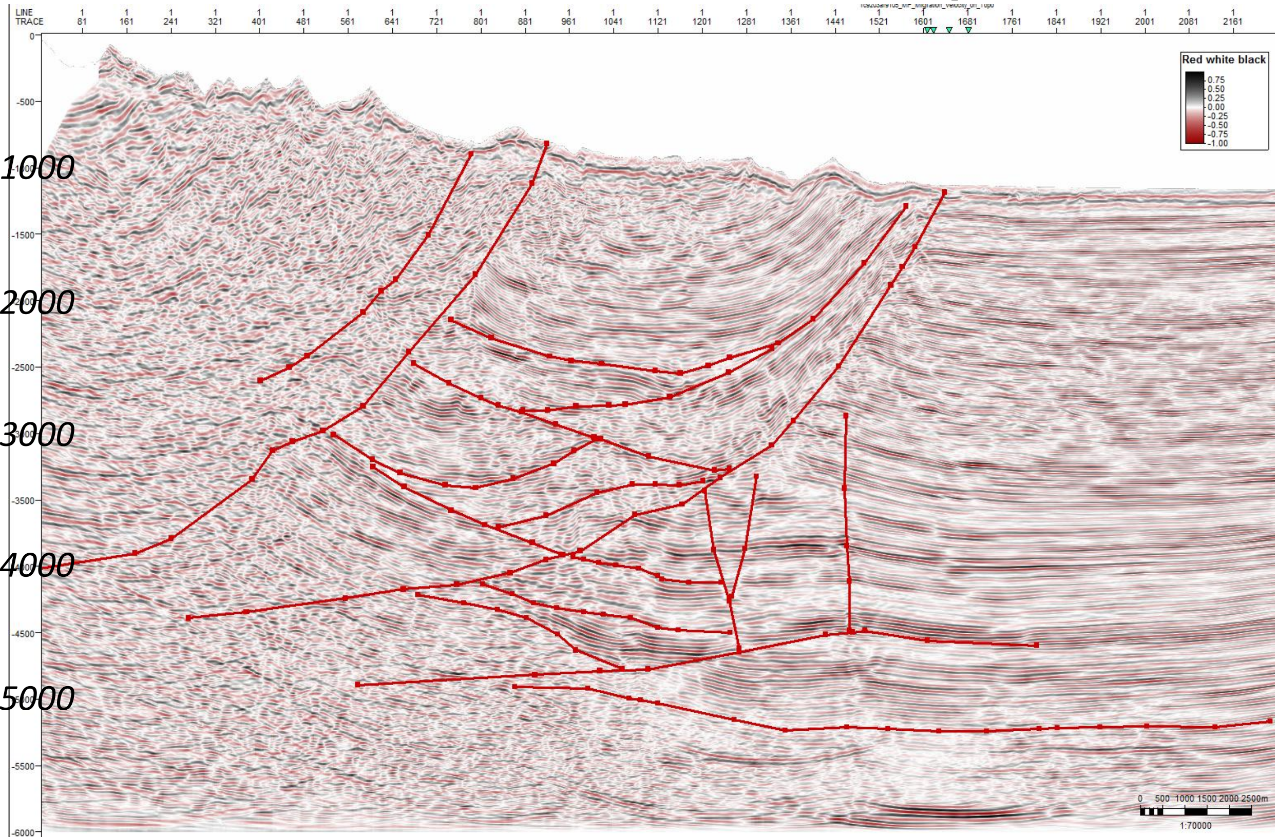
I Anexo: Sección sísmica Migrada y Pre-apilada en tiempo PSTM con interpretación geológica.
