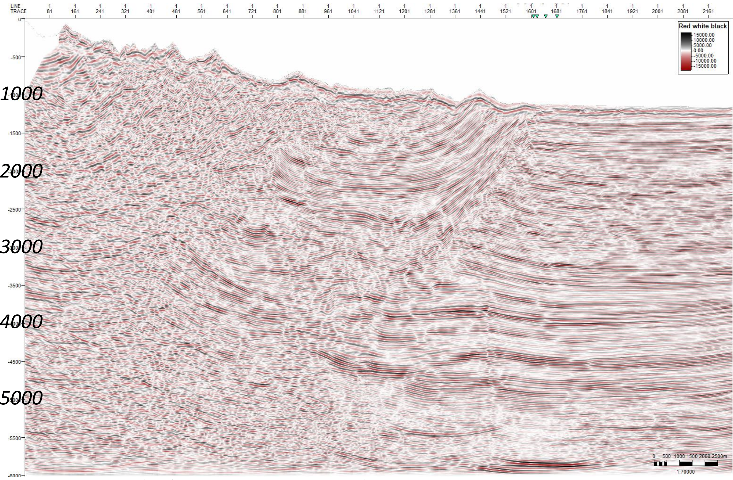
H Anexo: Sección sísmica Post Apilada Multifoco.
