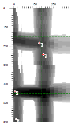
Ilustración 19. Columna 122 parte baja resultado inspección.
