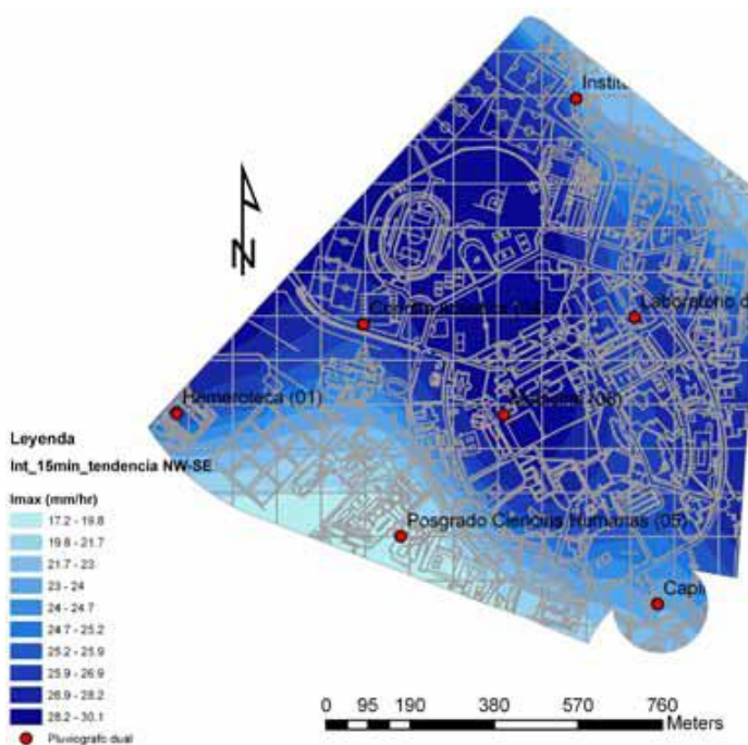
Ilustración 1. Intensidades máximas en 15 minutos fuente (Rodríguez et al., 2008)
