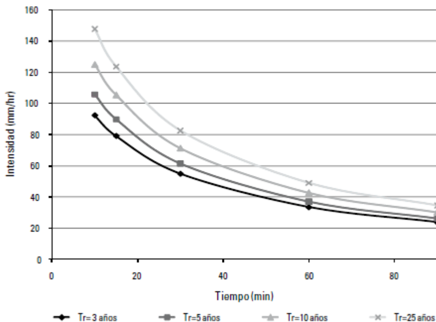
Ilustración 5. Curvas IDF Estación Hidrometeorológica Universidad Nacional de Colombia. Fuente Acueducto (Rodríguez et al., 2008).
