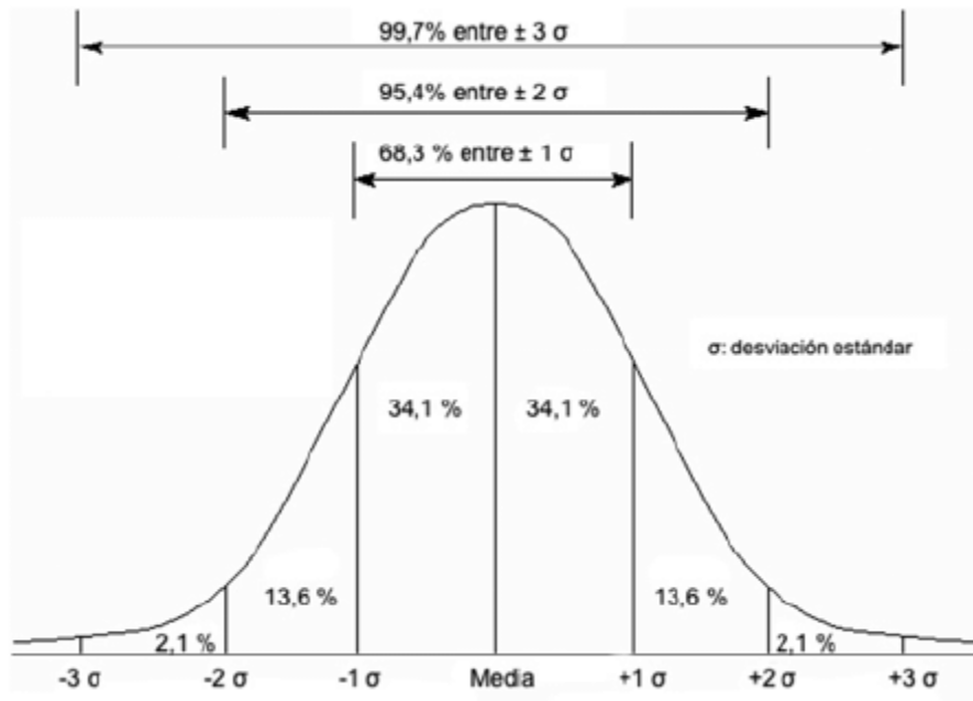
Ilustración 9. Distribución Normal.
