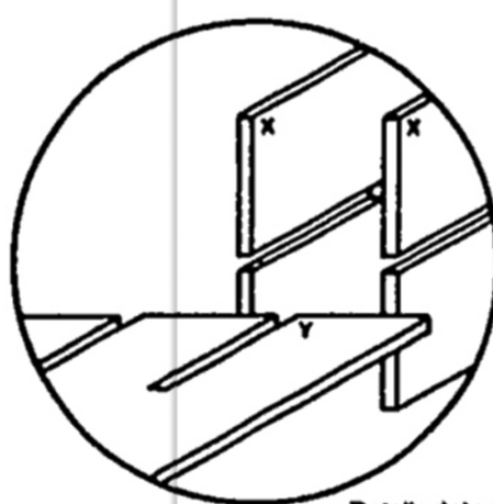
Detalle del ensamble para formar la cuadrícula para botellas acostadas
