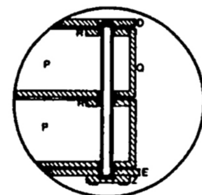
Detalle mecanismo para los cajones abatibles
