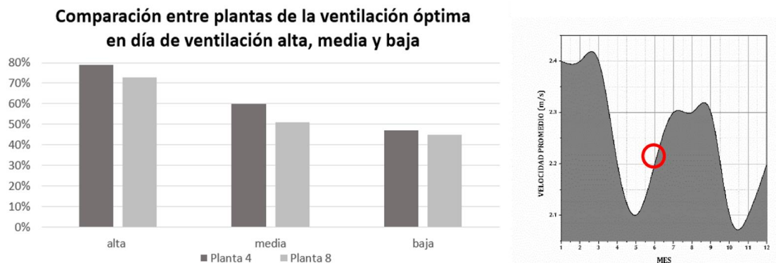
Figura 6 - Izquierda: Eficiencia de ventilación natural de los dos pisos del edificio de la EDU en las tres fechas de análisis de junio. La eficiencia del 100% corresponde a un espacio que durante todo el tiempo de uso supera los niveles de renovación de aire de referencia. Derecha: Promedio mensual de velocidad de viento en Medellín. Se resalta junio, con una velocidad media cercana al promedio anual. Fuente: Atlas del Viento de Colombia (IDEAM, 2017).
