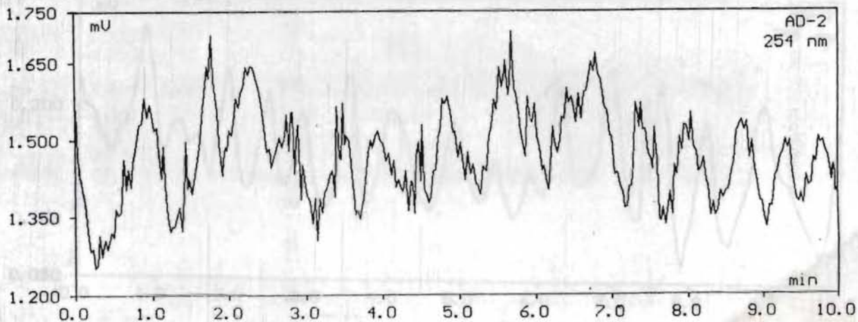
Cromatograma del ruido.
