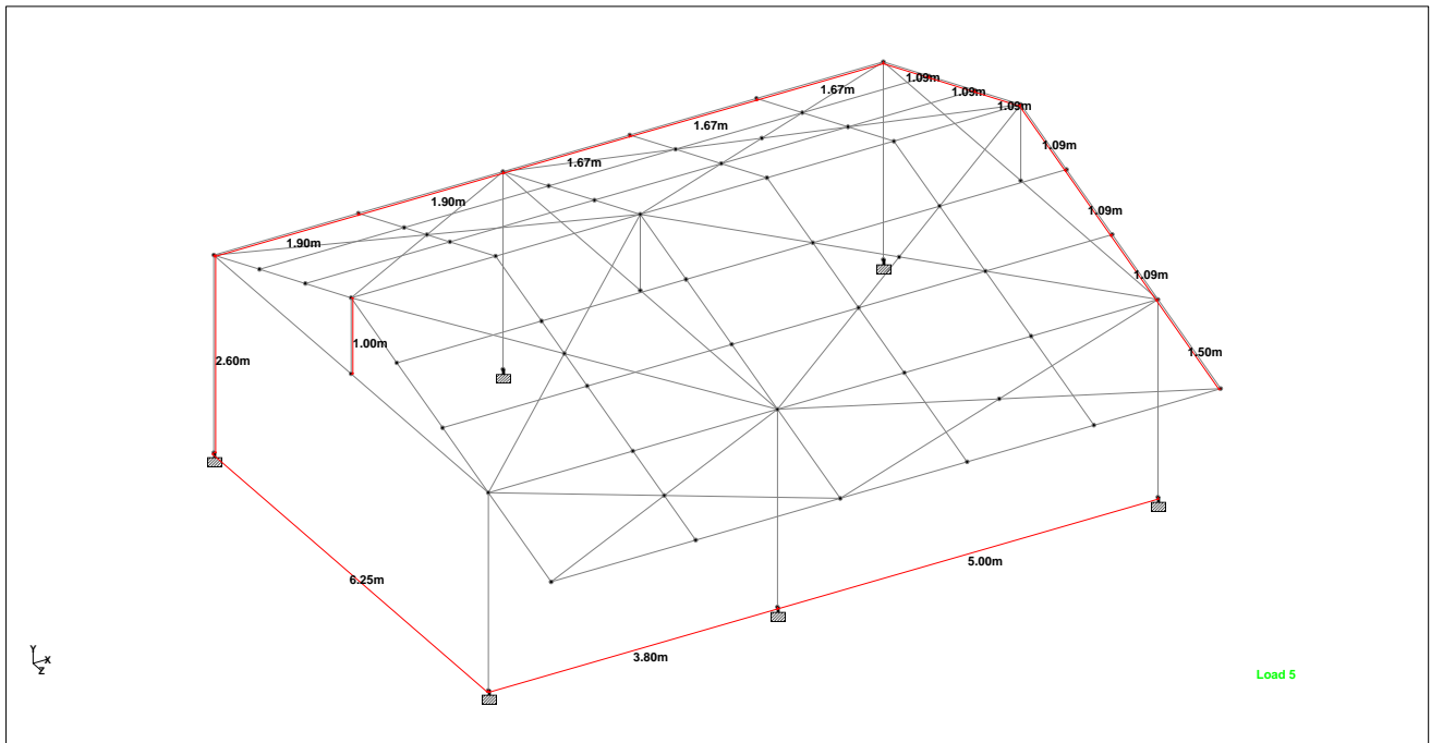
MEDIDAS MODELO AULA
