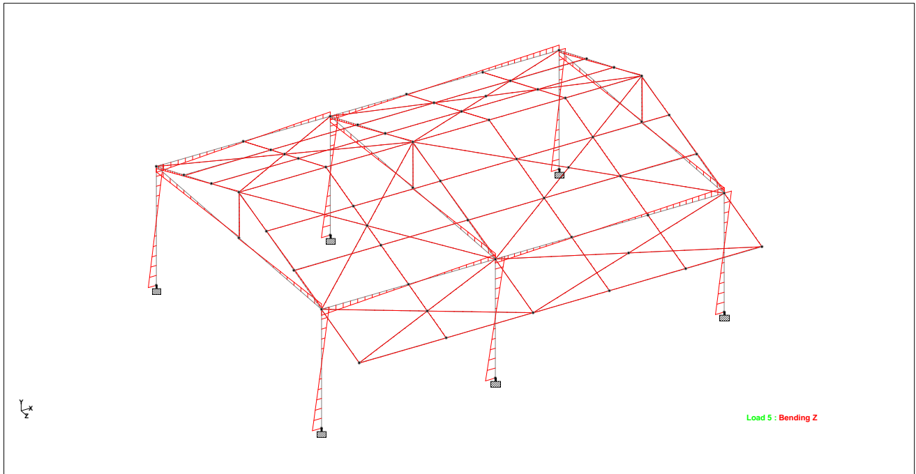
DIAGRAMA DE MOMENTOS EN Z MODELO GENERAL AULA
