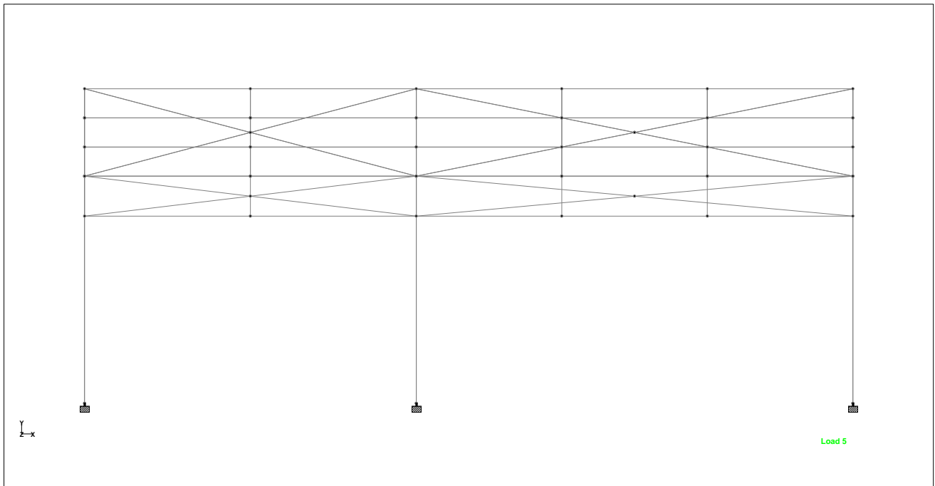
ALZADO FRONTAL MODELO AULA
