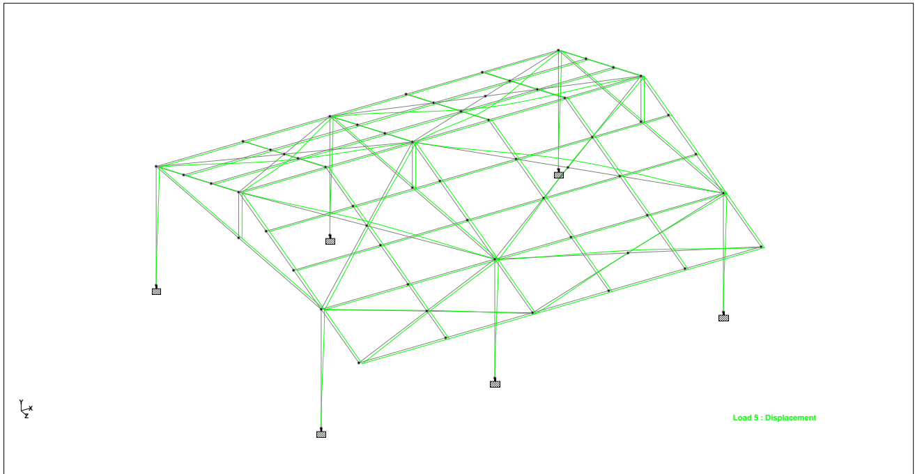
DIAGRAMA DE DSPLAZAMIENTOS MODELO GENERALL AULA
