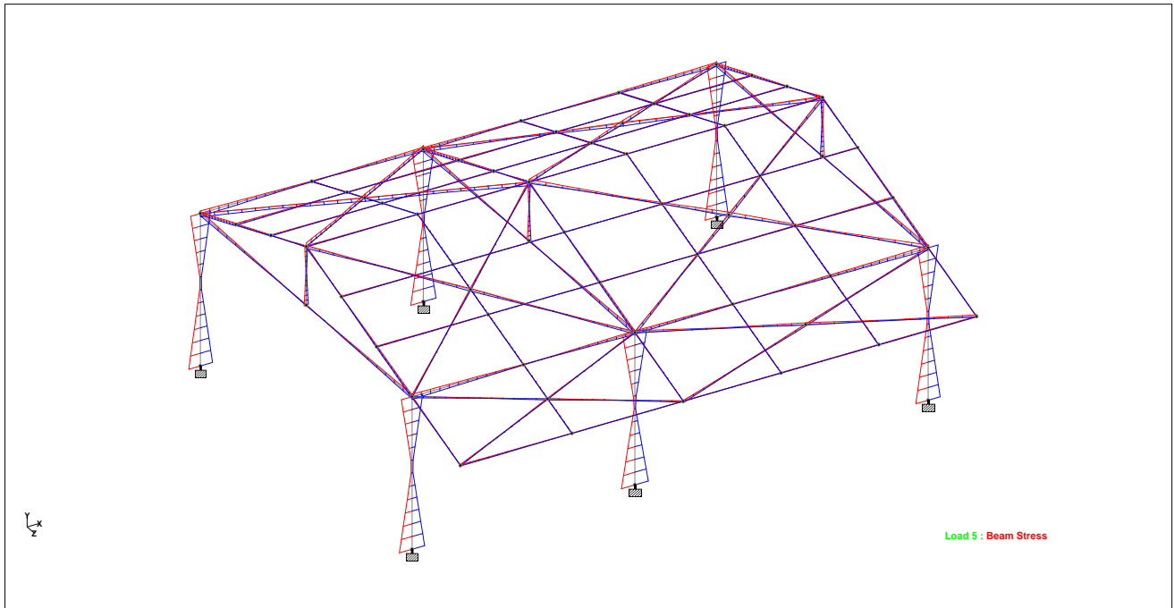
DIAGRAMA DE ESFUERZOS MODELO GENERAL AULA
