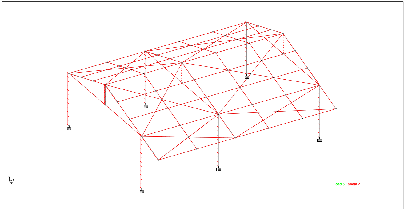
DIAGRAMA DE FUERZAS CORTANTES EN Z MODELO AULA
