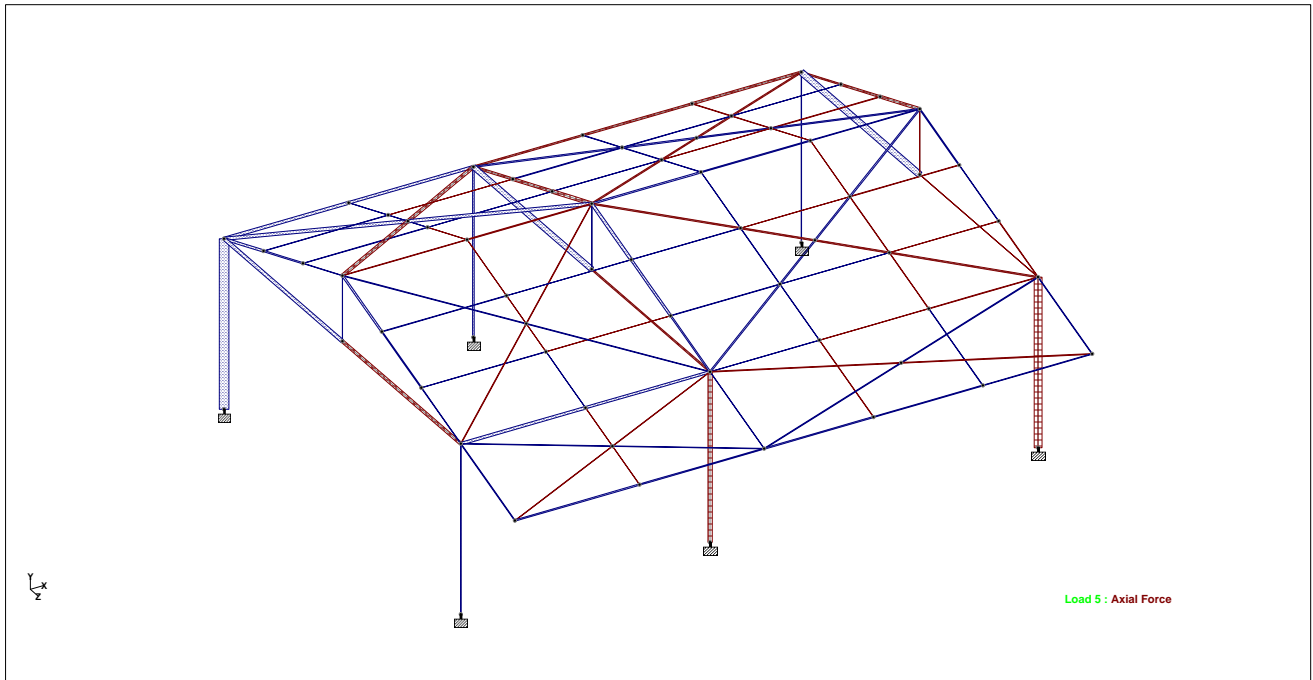
DIAGRAMA DE FUERZAS AXIALES MODELO AULA
