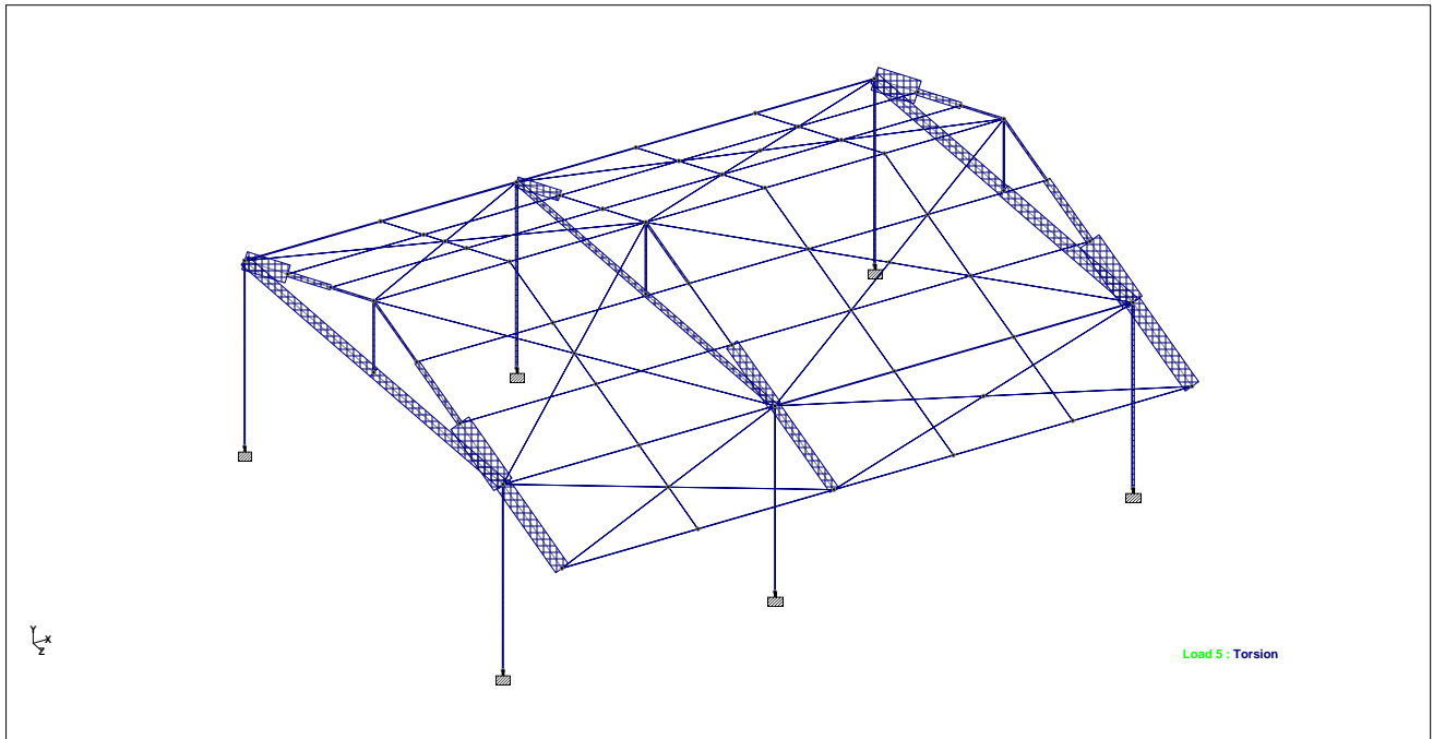
DIAGRAMA DE MOMENTOS TORSORES MODELO GENERAL AULA
