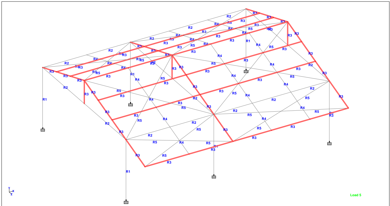
TUBULARES CUBIERTA 160X160X6 MM.
