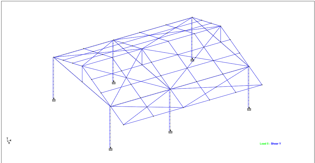
DIAGRAMA FUERZAS CORTANTES EN Y MODELO AULA
