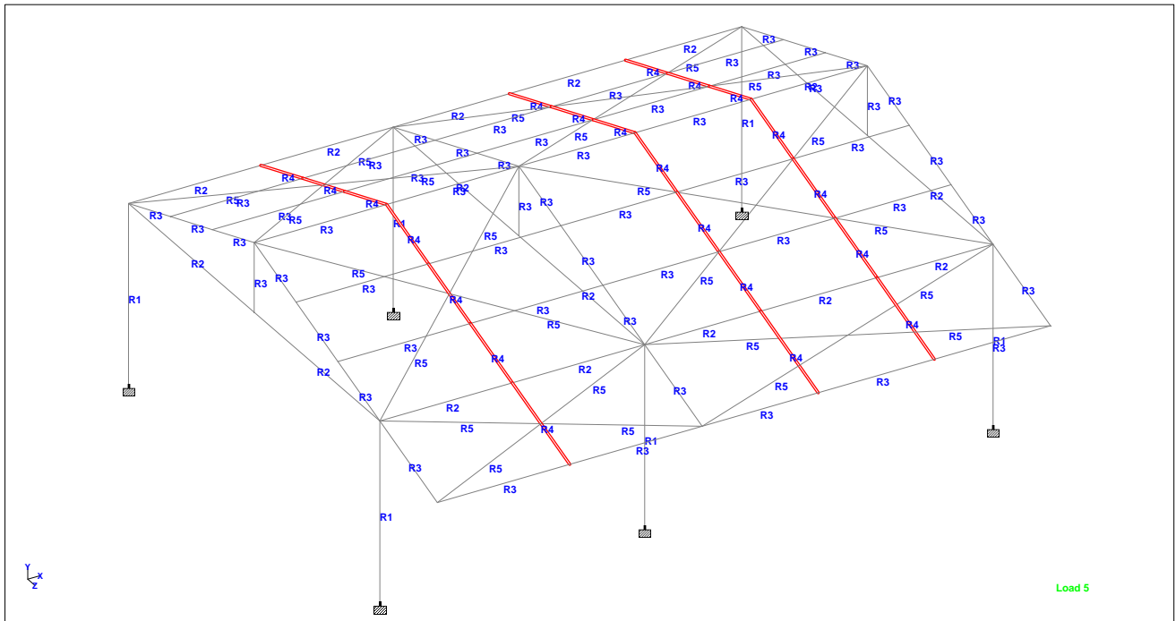
TIRANTILLOS VARILLA DE 3/8".
