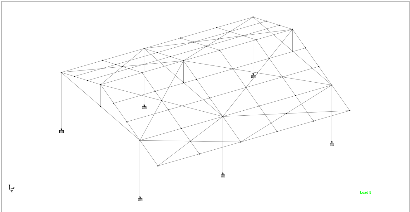
ISOMETRICO MODELO AULA
