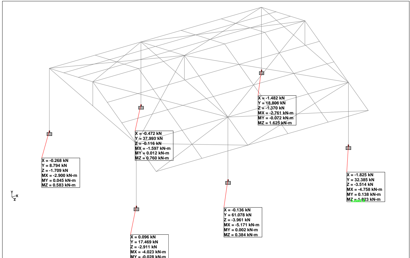
DIAGRAMA DE REACCIONES MODELO GENERAL AULA
