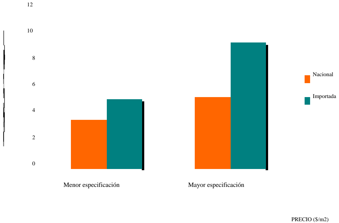
Figura 4.3. Comparación gráfica en precio para geomallas nacionales e importadas (LaFayette, 2002; Geosintec, 2002)
