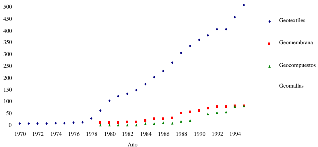
Figura 3.3. Distribución del mercado internacional de los geotextiles (FAO, 2001).
