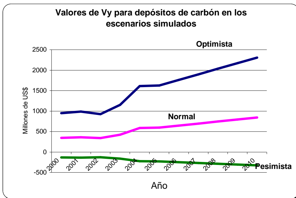
Figura 2: Valores de V_y para depósitos de carbón en los escenarios simulados
