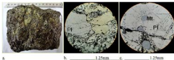
Pentlandita (Fe, Ni) 9 S 8 , Falconbridge Mine, distrito de Sudbury, Ontario Canadá. a: Muestra de mano, b. sección pulida, nicoles paralelos. Pentlandita(Pl), pirita(Pi), calcopirita(Cp). c. Sección pulida, nicoles paralelos. pentlandita (Pl), magnetita (Mt).
