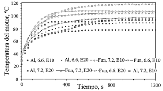
Figura 17. Histórico de temperaturas del motor durante el calentamiento. Fuente: Los autores.
