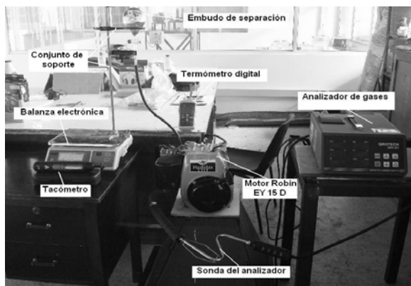
Figura 1. Configuración experimental.
