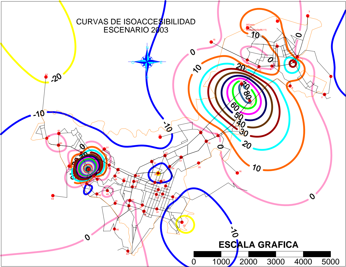
Figura 20. Ganancia y Pérdida en Tiempos de Accesibilidad
