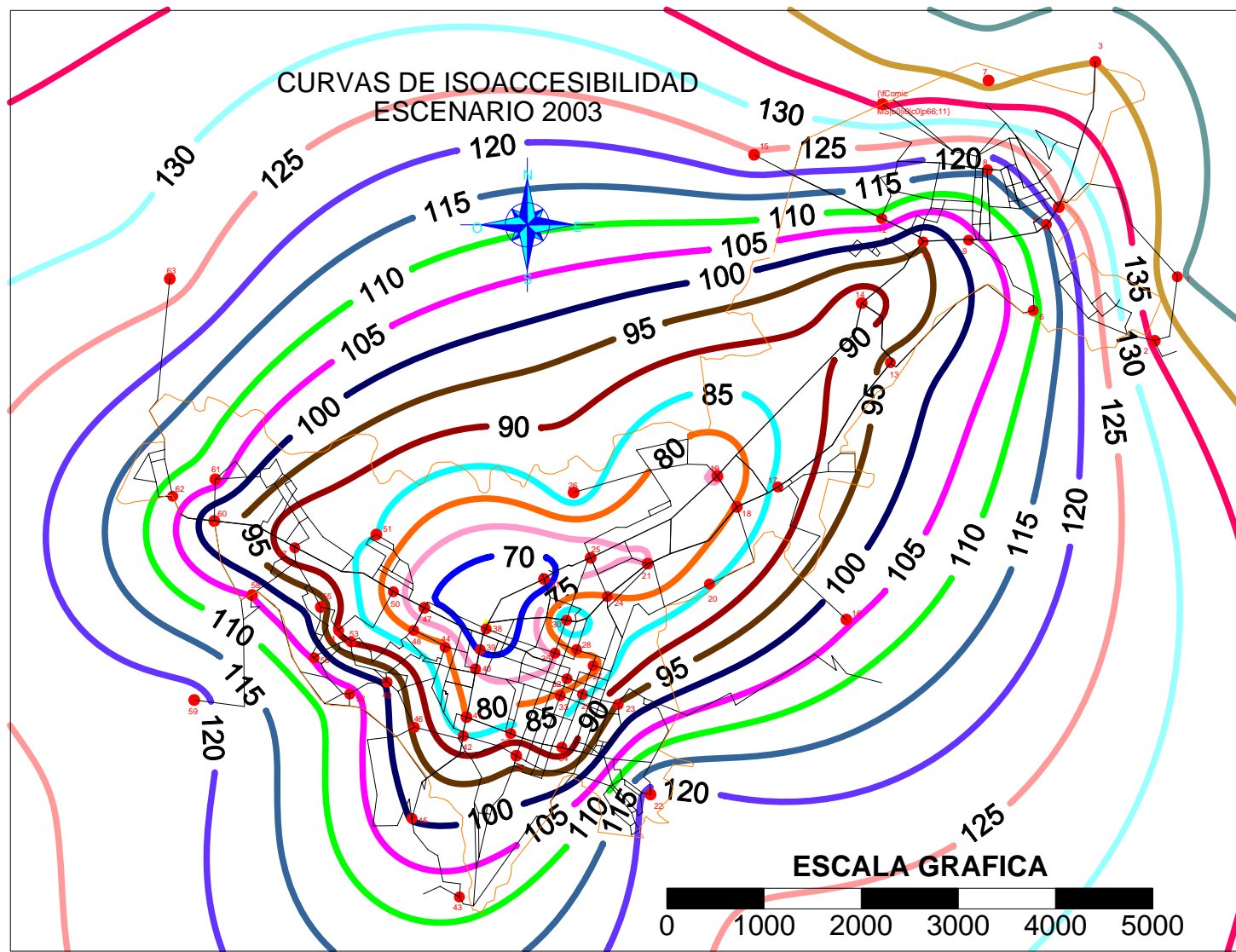
Figura 19. Curvas de Isoaccesibilidad, 2003
