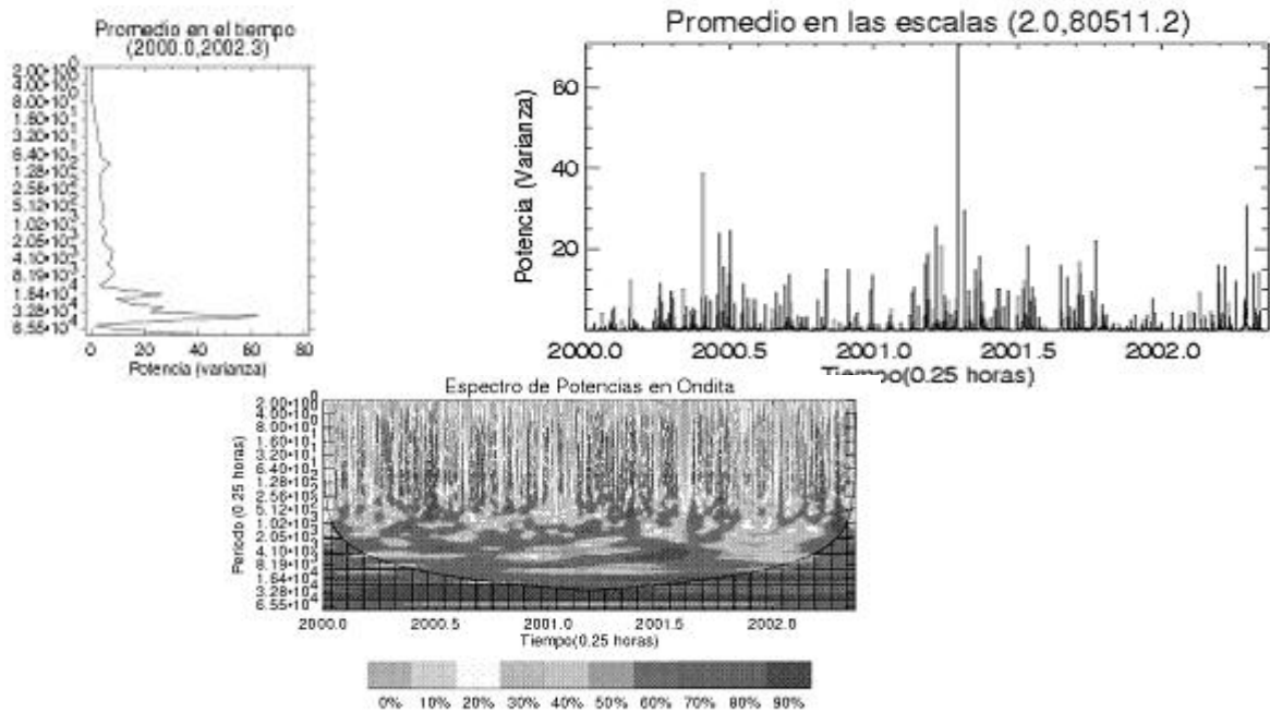
FIGURA 7. Estación Santa Rita intervalo 15 minutos a) Promedio en el tiempo, b) Promedio en las escalas, c) Espectro de potencias.
