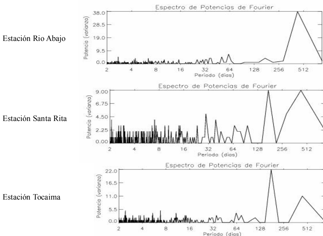
FIGURA 5. Continuación. Espectro de potencias (FFT) para las series diarias de las estaciones Bizcocho, Corrientes, el Peñol, Río Abajo, Santa Rita y Tocaima.
