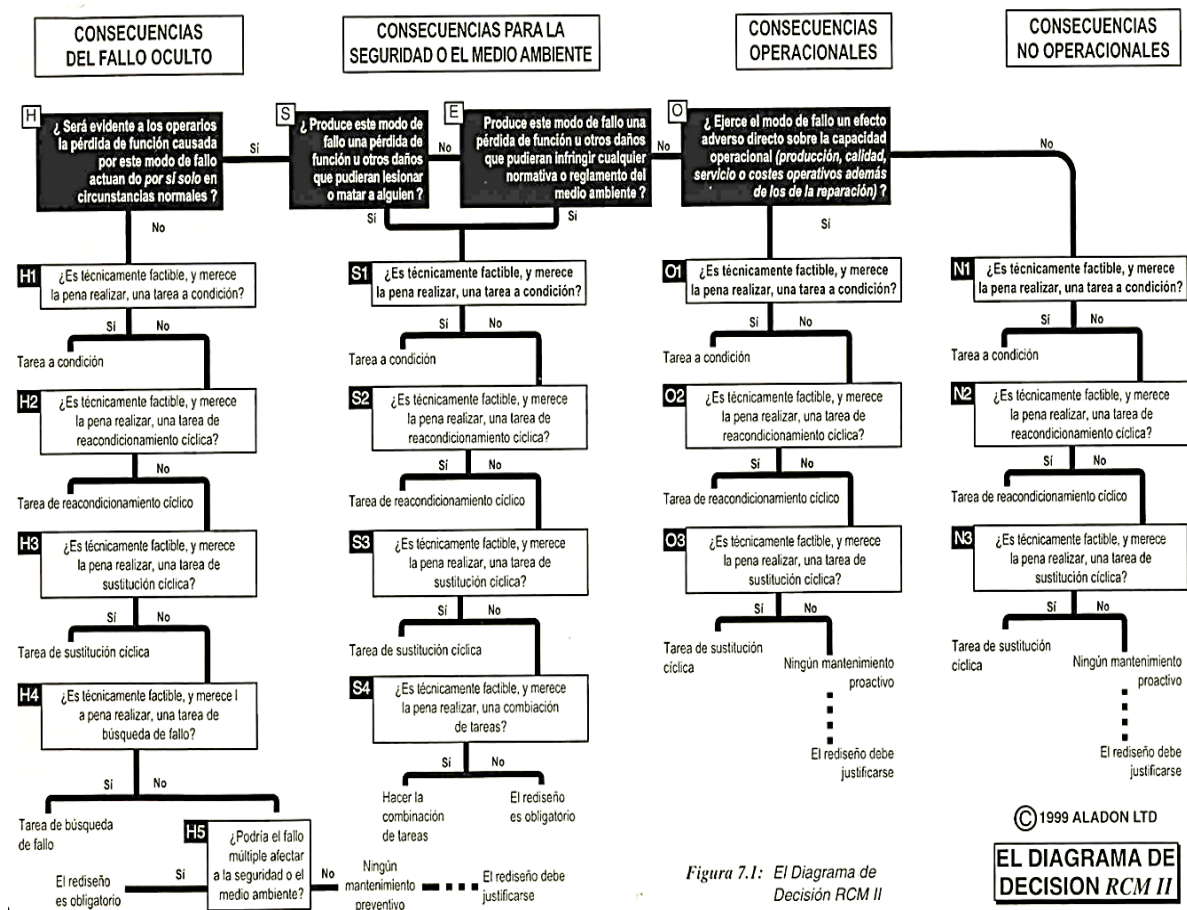
Figura 25. Diagrama de decisión de actividades de mantenimiento RCM II
