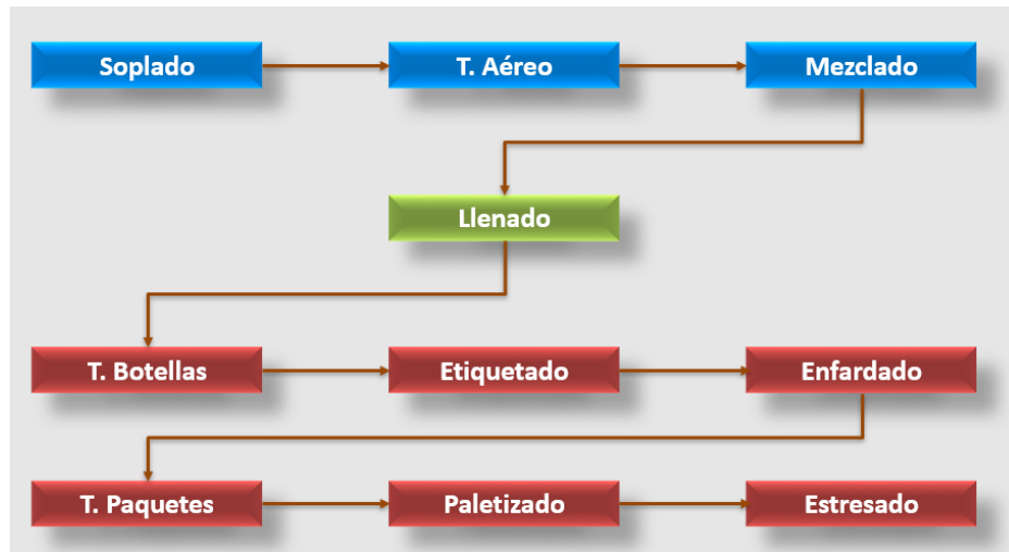
Figura 9. Distribución típica de una línea de producción de embotellado
